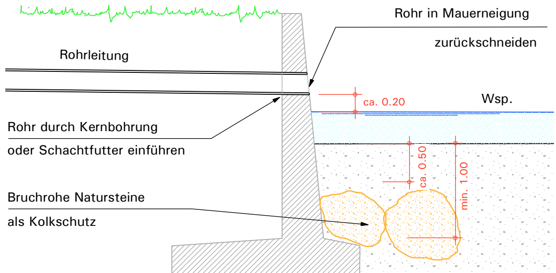
Querschnitt 1:50
