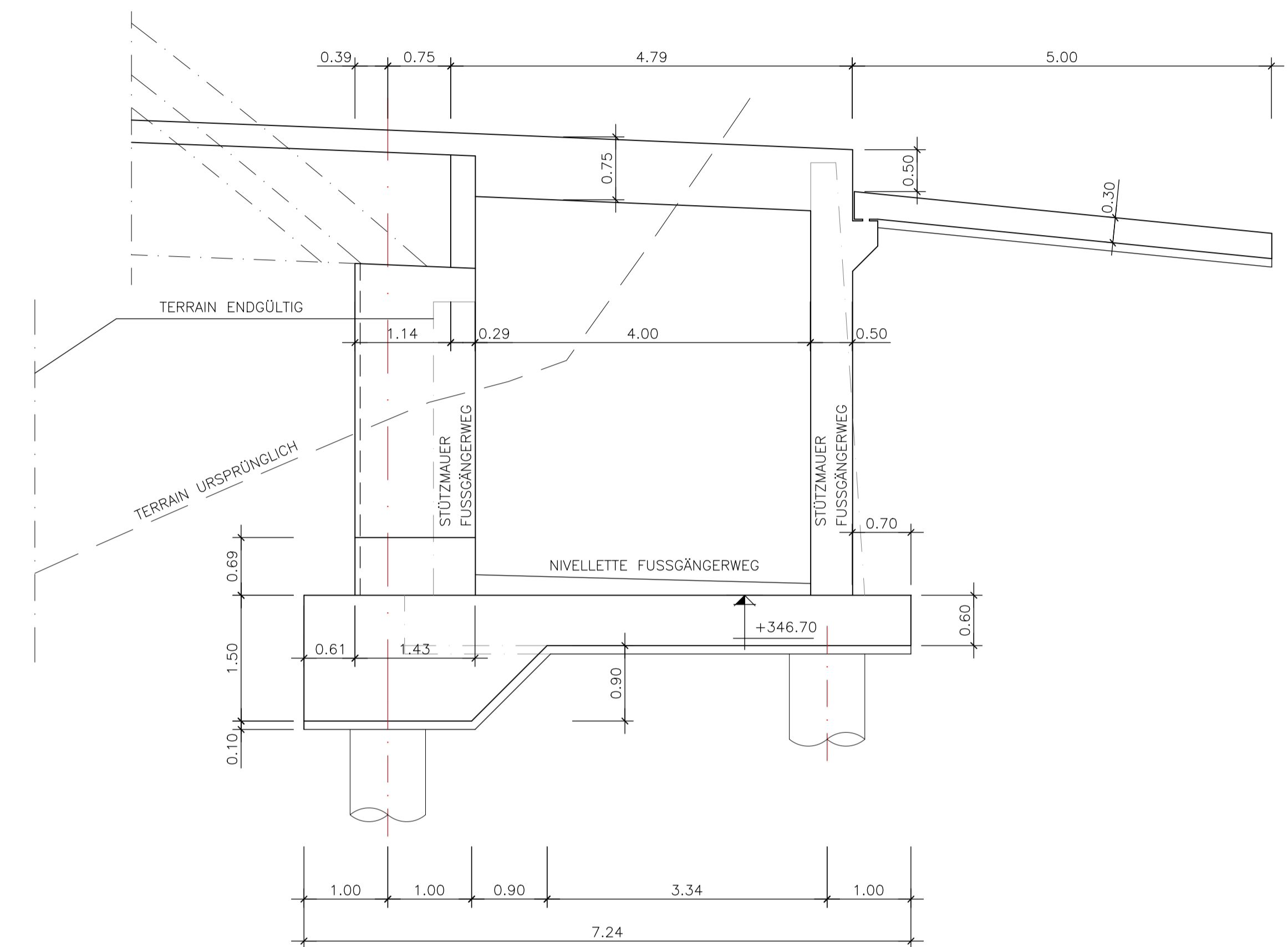
ANSICHT B 1:50
