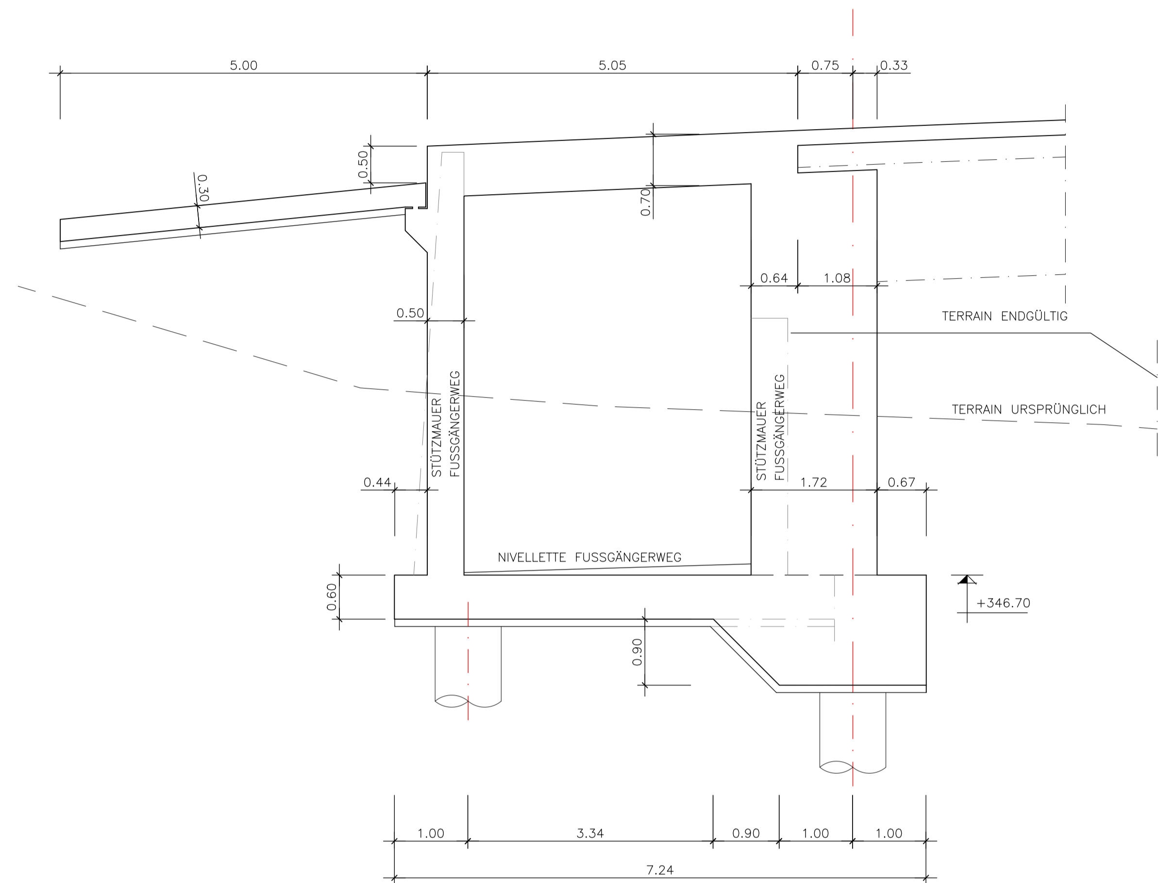
ANSICHT A 1:50
